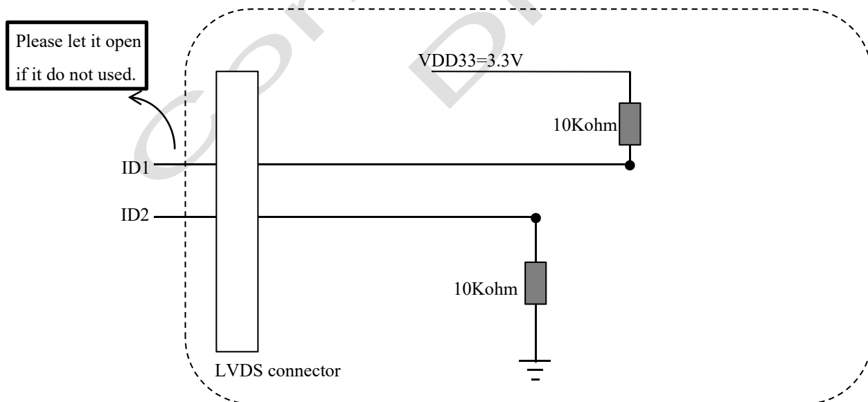
Fig. 4.2 ID1/ID2 set
